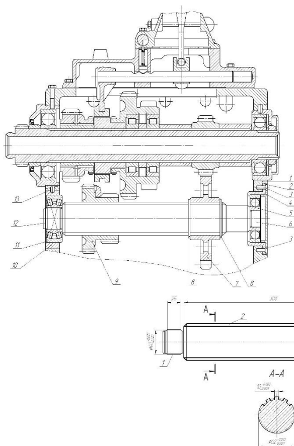
Рисунок 2 – Эскиз вала заднего хода
